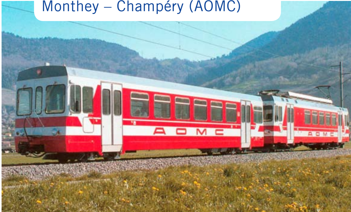
Pendelzug der AOMC mit dem von PROSE entwickelten Steuerwagen
